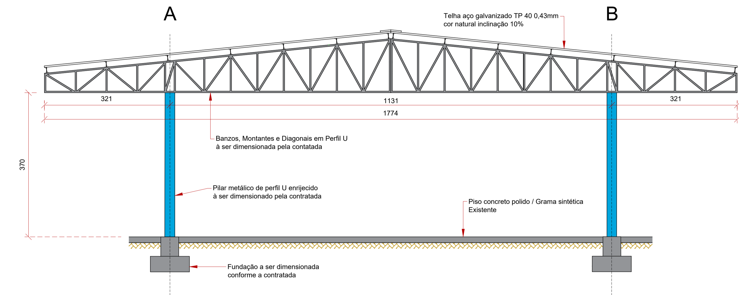
EIXO 1-3 QUADRA COBERTA ESC.: 1/50
