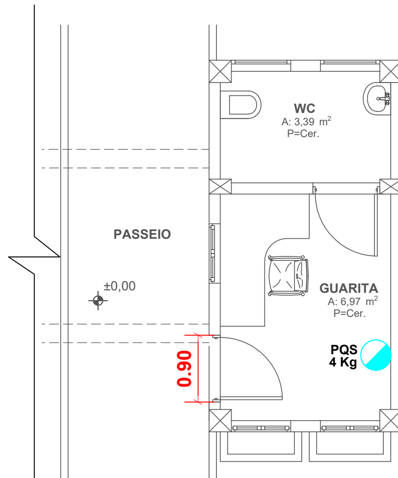
PLANTA BAIXA ÁREA: 44,20m² ESC.: 1/50
