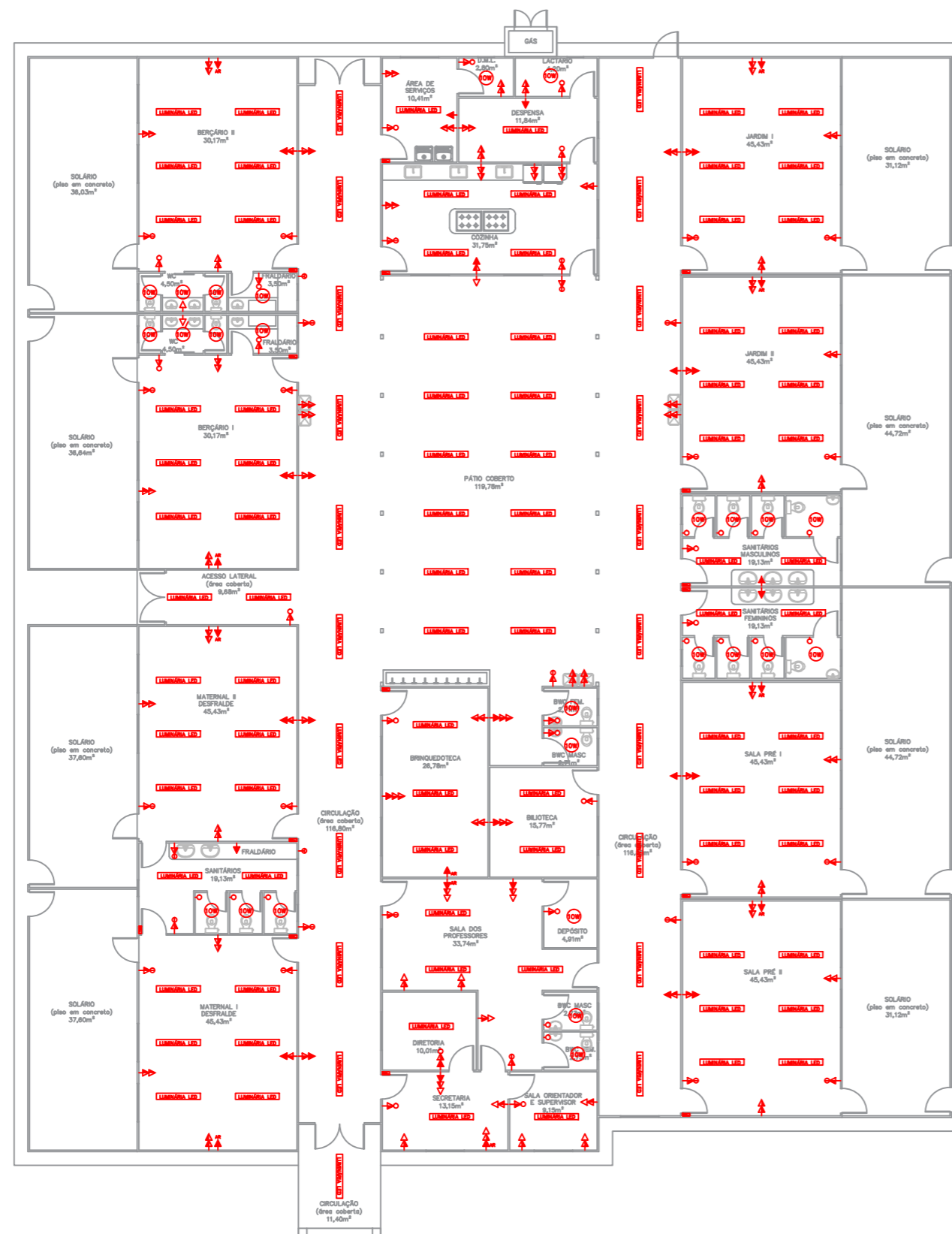
PLANTA BAIXA – ELÉTRICO Esc. 1/50
