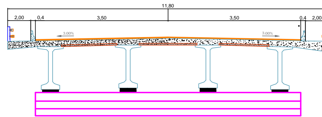
CORTE TRANSVERSAL ESC.: 1/200
