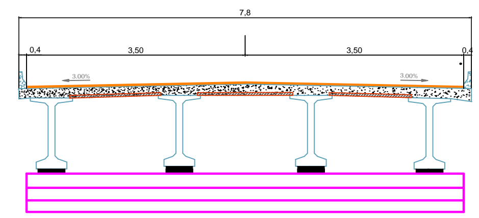
CORTE TRANSVERSAL ESC.: 1/200
